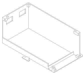
Korpus podstawy - prawy
