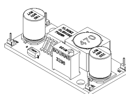
Przetwornica step-down LM2596
